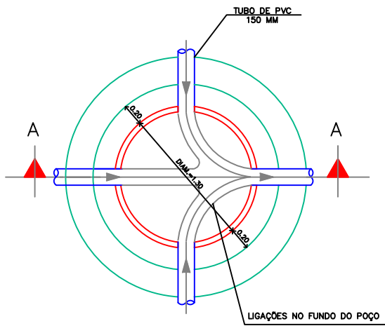
PLANTA – Poço de Visita em Aduelas de Concreto ESCALA 1:20
