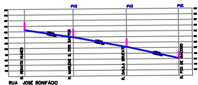
PERFIL DAS RUAS ESCALA 1:1000
