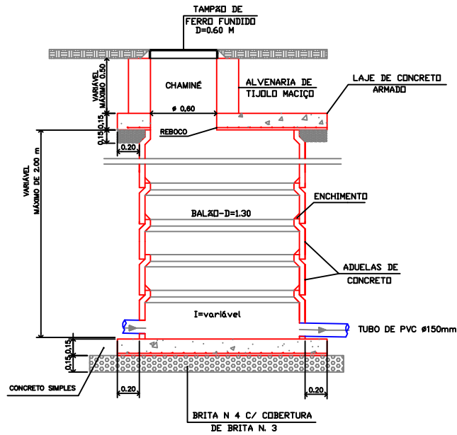
CORTE AA – Poço de Visita em Aduelas de Concreto ESCALA 1:20
